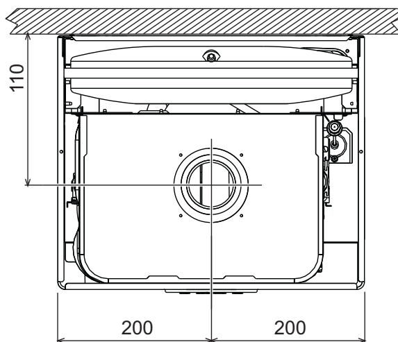
fig. 49 - Vista dall'alto
