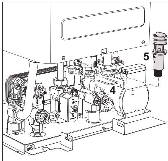
fig. 42 - Flussometro
