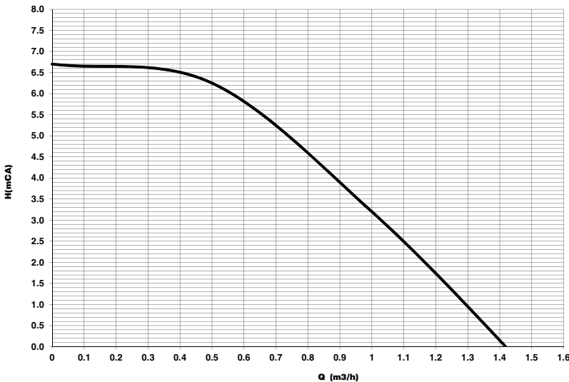
fig. 62- Carga hidrostática residual disponible en la instalación
