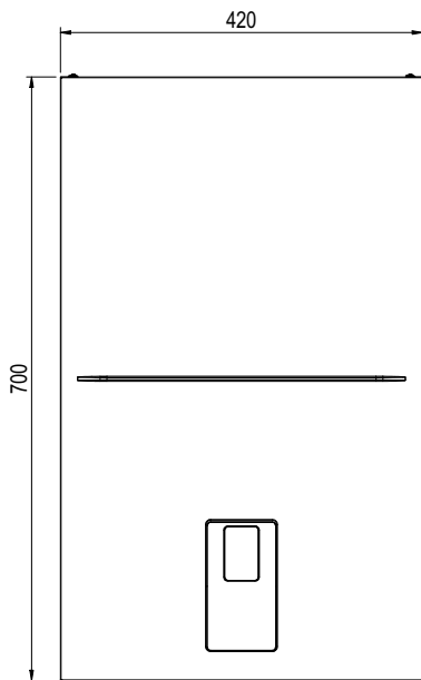
fig. 56- Vista frontal
