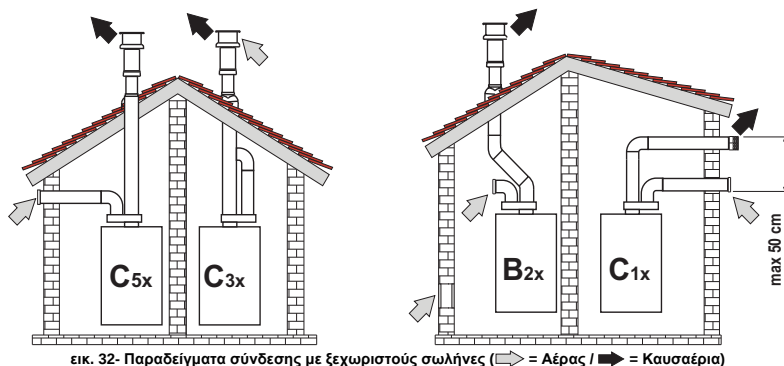
εικ. 32- Παραδείγματα σύνδεσης με ξεχωριστούς σωλήνες (⇐ = Αέρας / ➡ = Καυσαέριο)
