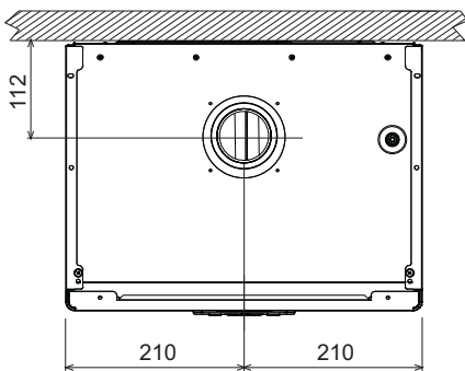
εικ. 58- Κάτοψη
