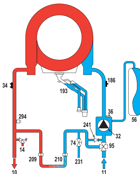
fig. 61- Circuitul hidraulic
