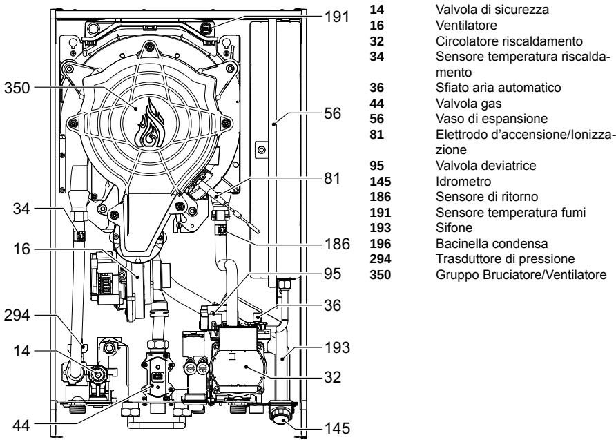
fig. 60 - Vista generale
