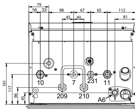
fig. 59- Vista inferior
