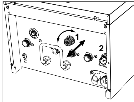
εικ. 26- Διακόπτης πλήρωσης
