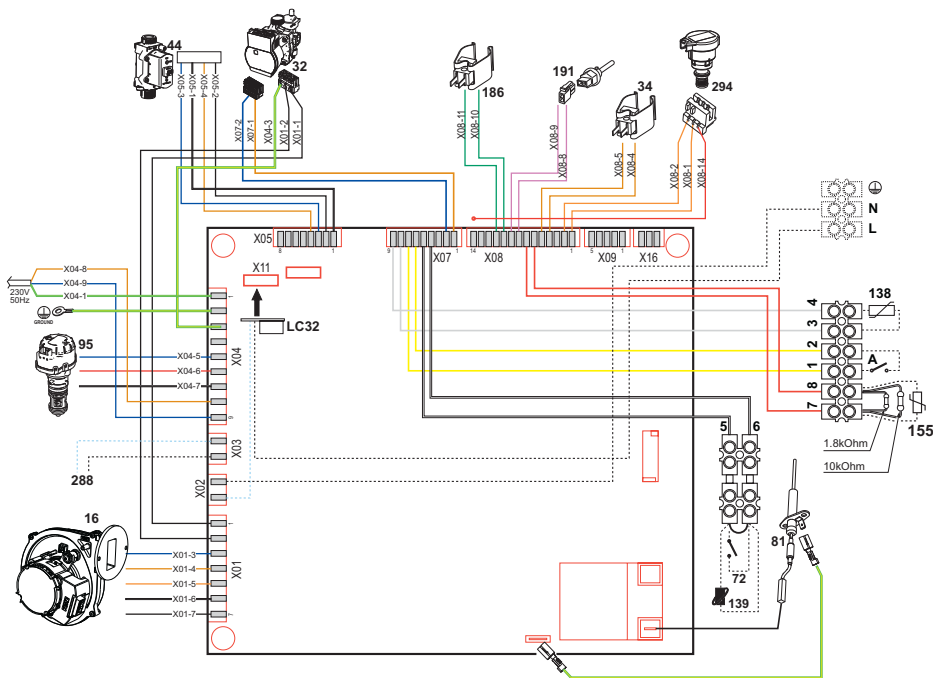
fig. 64- Schema electrică
