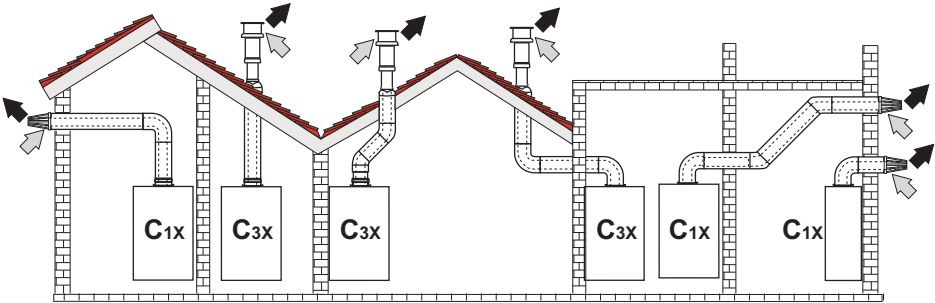
fig. 30- Ejemplos de conexión con tubos coaxiales (⇨ = aire / ⇨ = humos)
