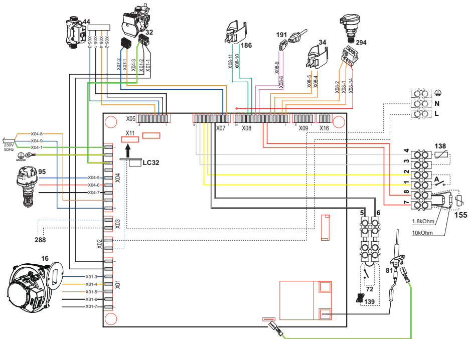
fig. 64- Wiring diagram
