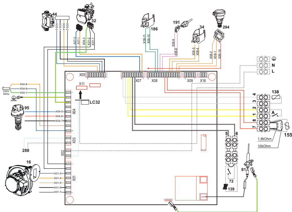
εικ. 64- Ηλεκτρολογικό διάγραμμα
