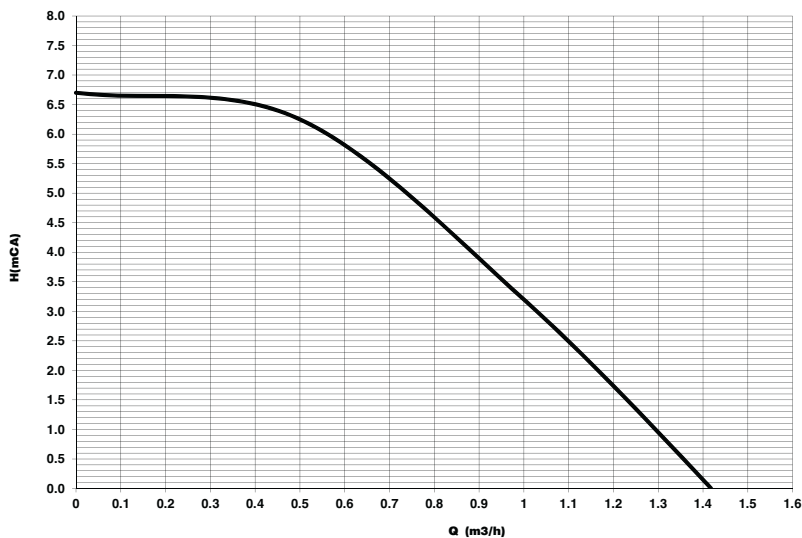
εικ. 62- Διαθέσιμο υπολειπόμενο μανομετρικό ύψος στην εγκατάσταση
