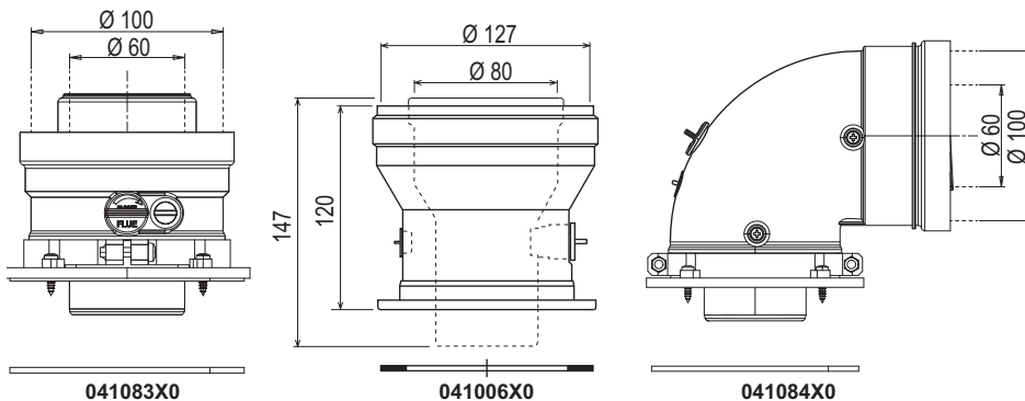
fig. 31- Accesorii de pornire pentru conducte coaxiale
