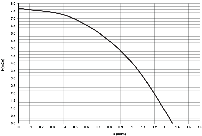
fig. 63 - Prevalenza residua disponibile all'impianto
