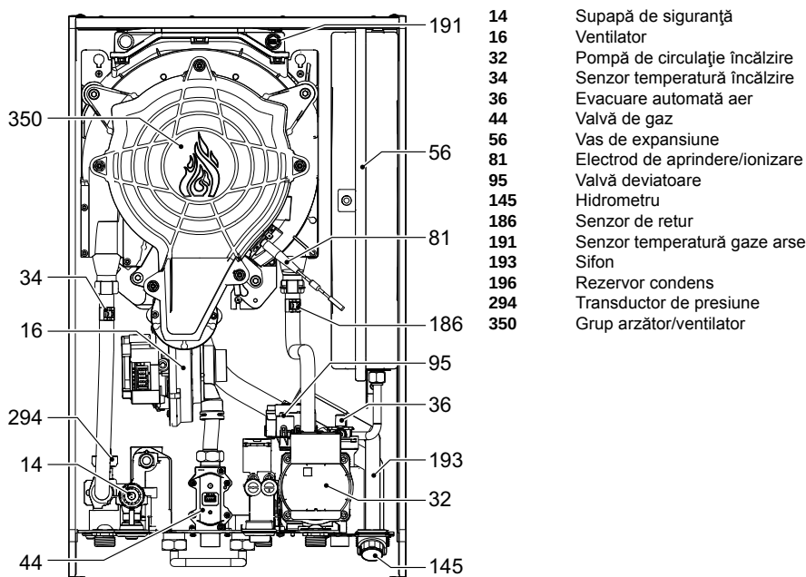
fig. 60- Vedere generală
