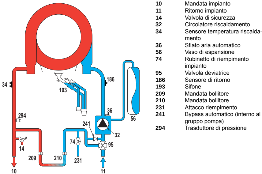
fig. 61 - Circuito idraulico
