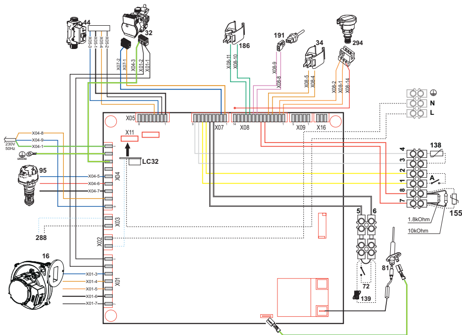
fig. 64 - Schema elettrico
