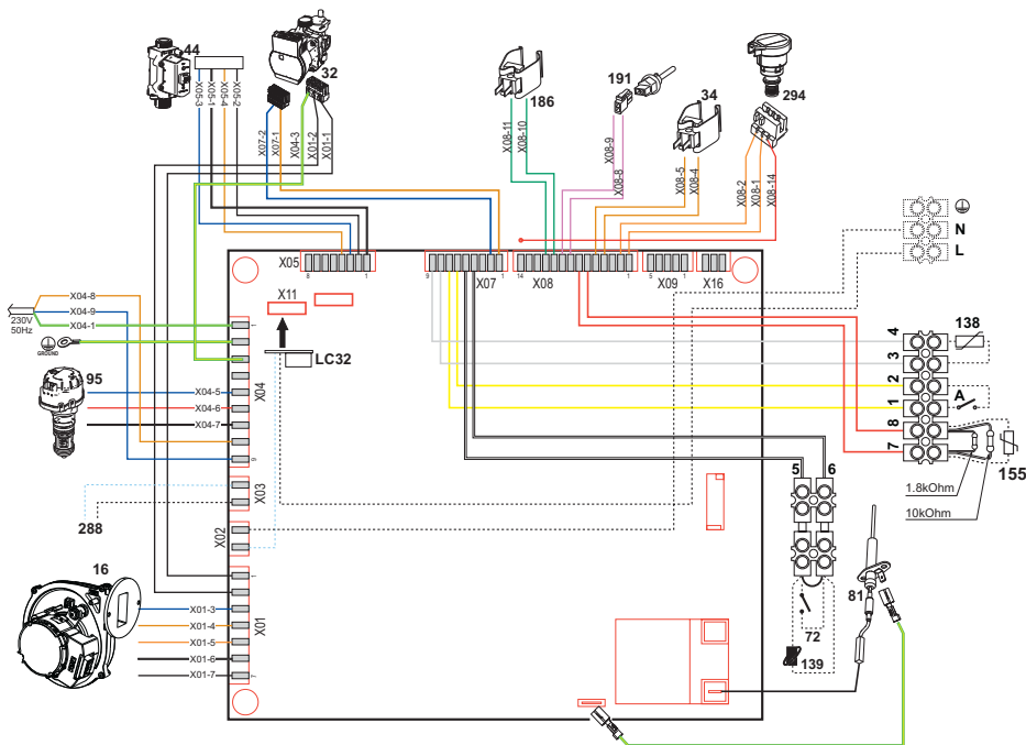
fig. 64 - Esquema eléctrico
