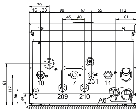
εικ. 59- Άνοψη
