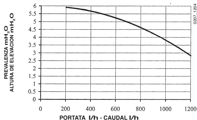
LUNA 280 i - 310 Fi
