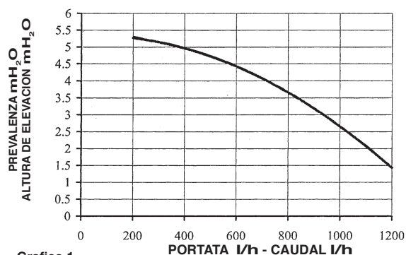
LUNA 240 i - 240 Fi
