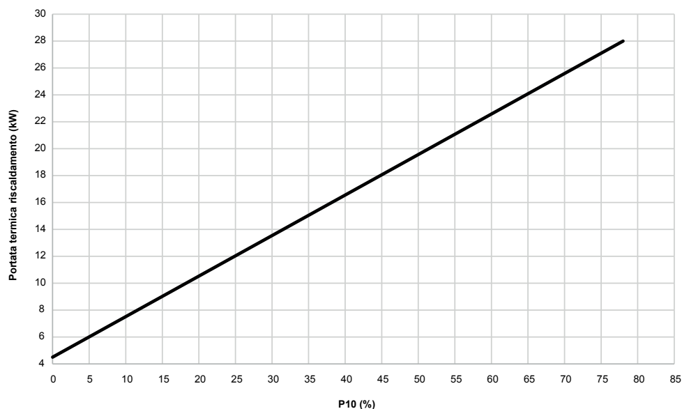
KALDAIA 28/35 G20 Curva P10 - Portata Termica Riscaldamento
