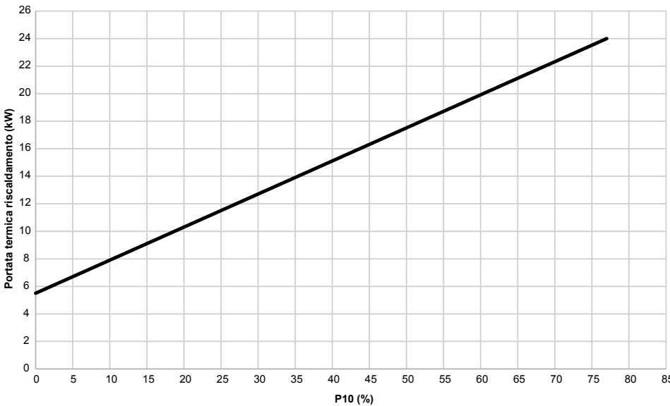
KALDAIA 24/30 G31 Curva P10 - Portata Termica Riscaldamento
