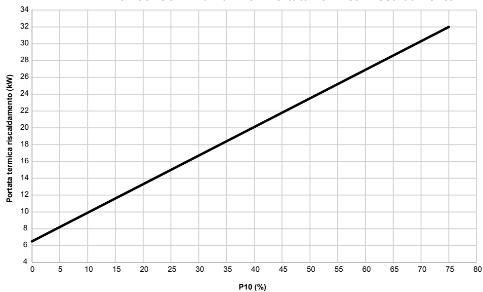
KALDAIA 32/35 G31 Curva P10 - Portata Termica Riscaldamento
