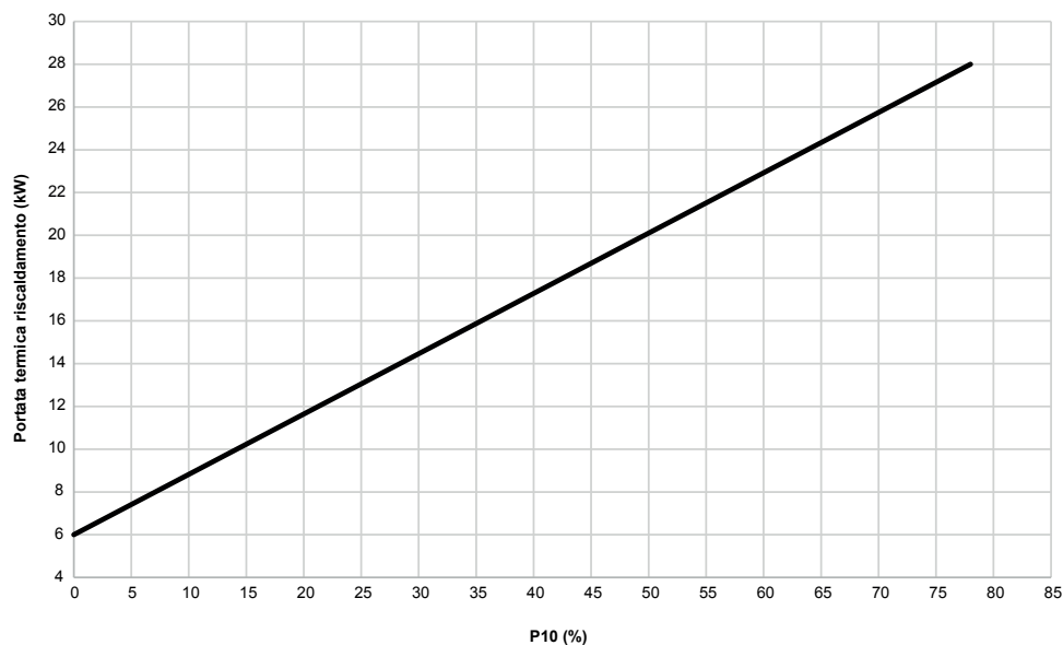
KALDAIA 28/35 G31 Curva P10 - Portata Termica Riscaldamento
