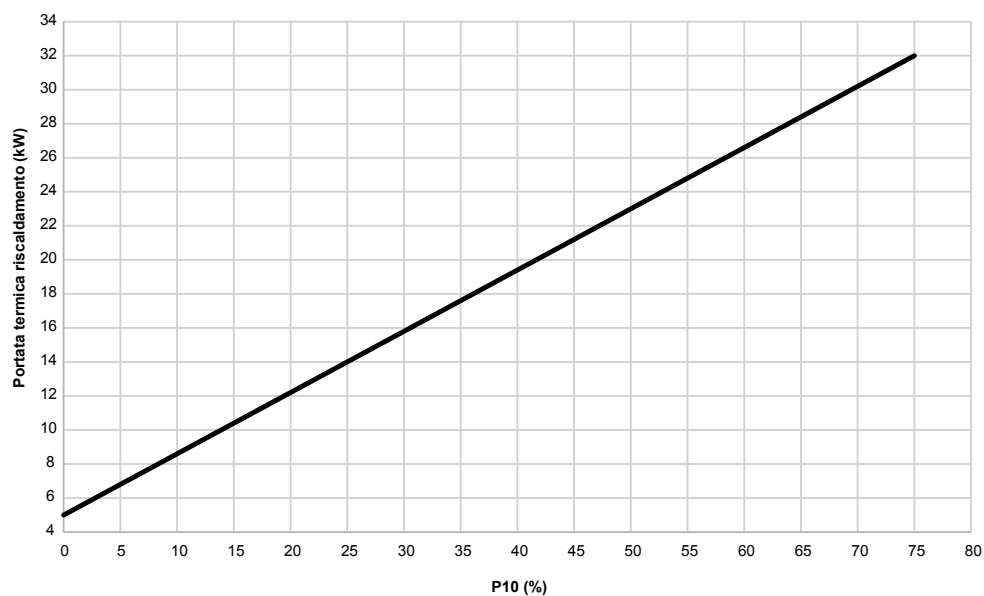
KALDAIA 32/35 G20 Curva P10 - Portata Termica Riscaldamento
